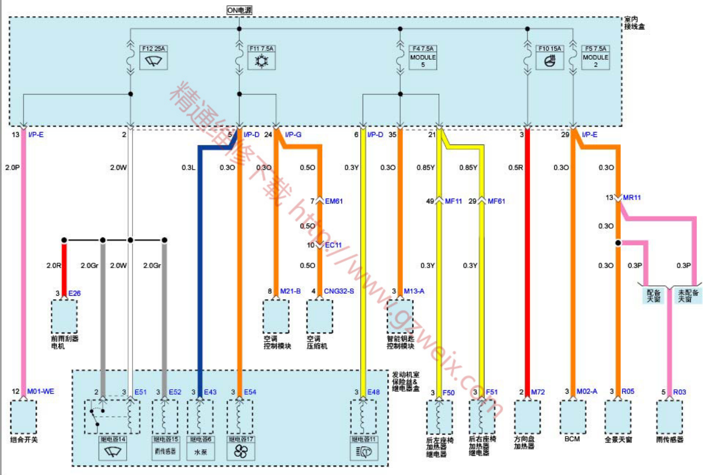
室内保险丝分布(2)
